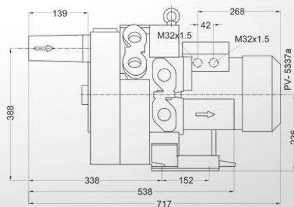
Dimensiones
